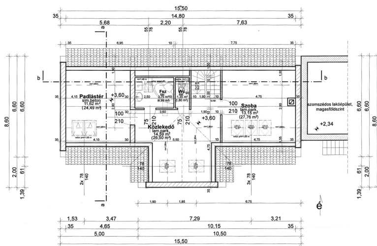
tetőtérszinti alaprajz, m=1:100 nettó alapterület: 44,46 m 2 (85,54m 2 )
