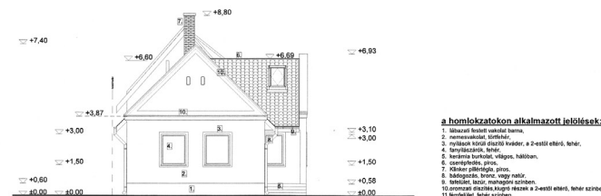
nyugati homlokzat, m=1:100
