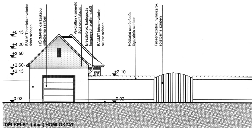
DELKELETI (utcai) HOMLOKZAT
