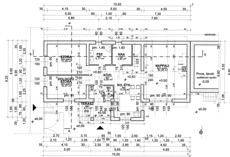
földszinti alaprajz, m=1:100 nettó alapterület: 82,78 m 2
