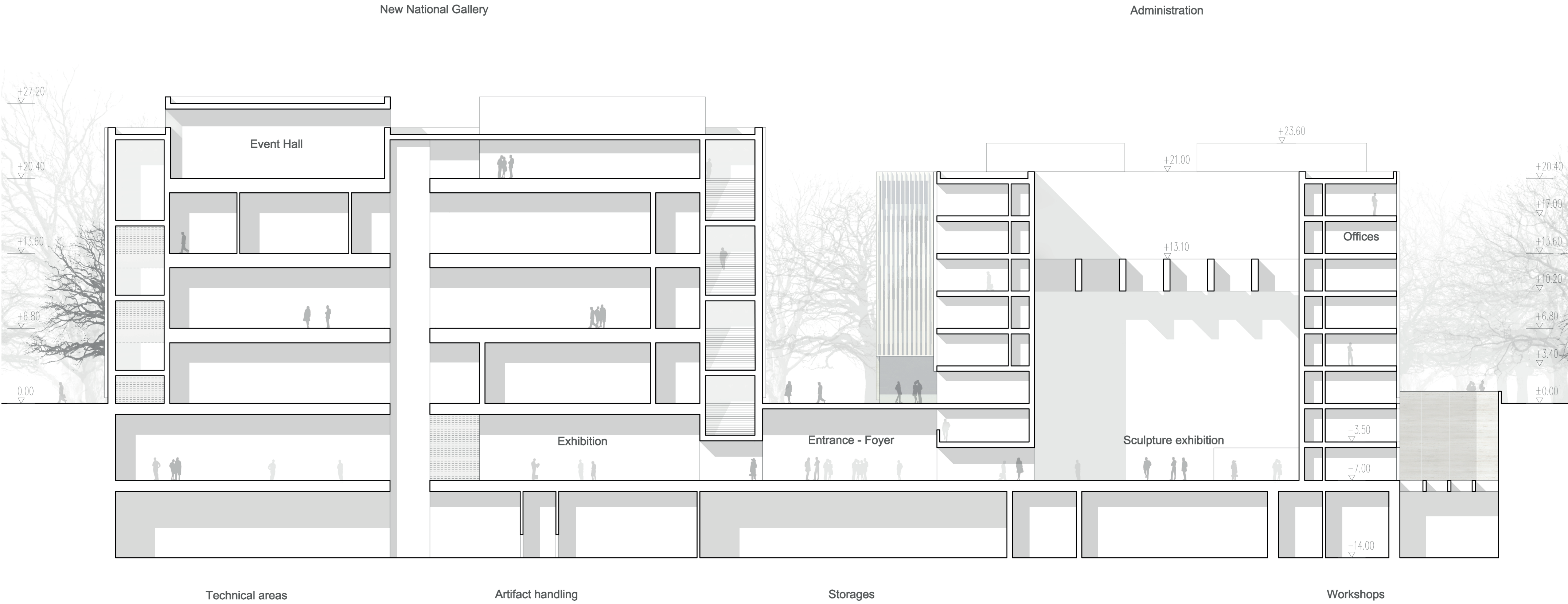
Section BB 1:250
