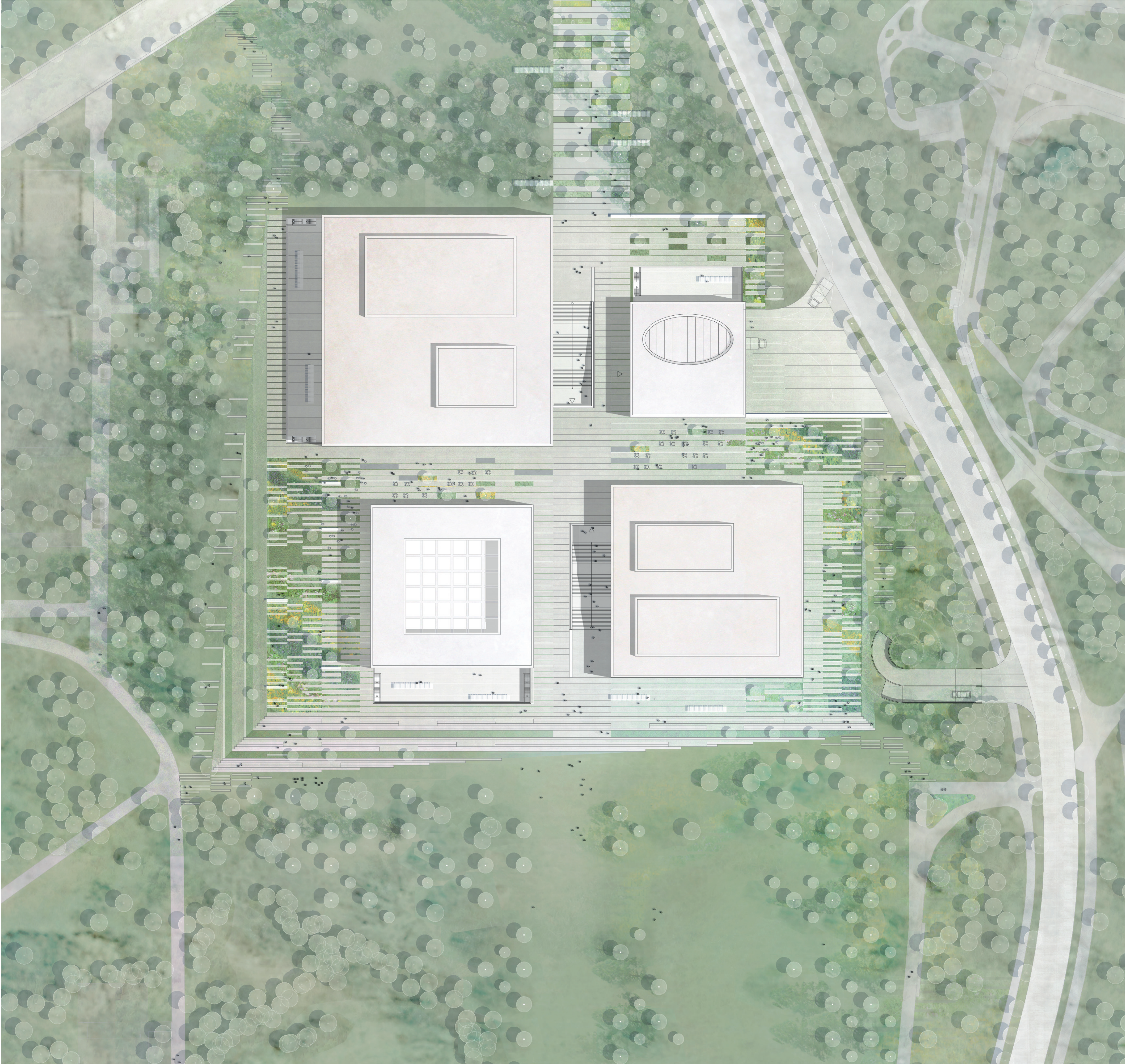
Siteplan 1:500
