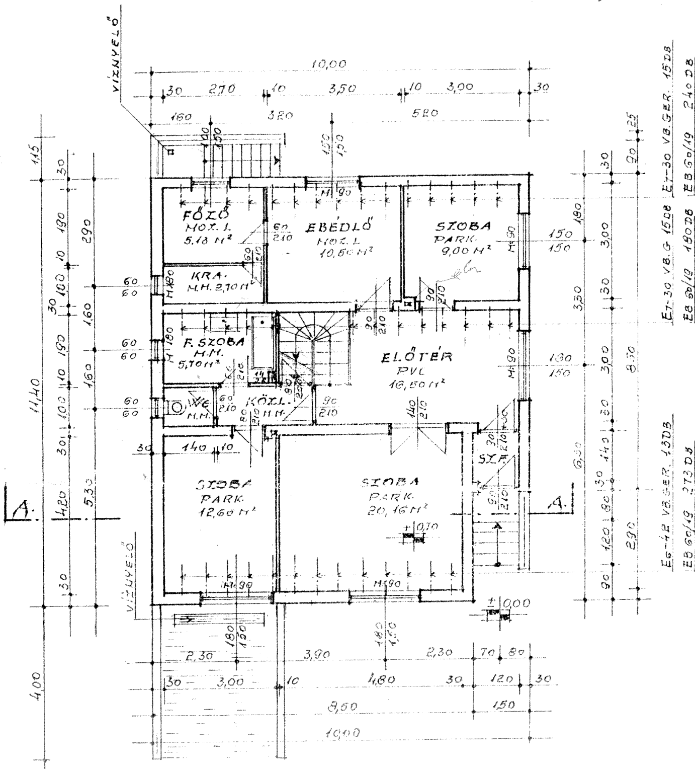
FSZ. ALAPRAJZ M 1:100
